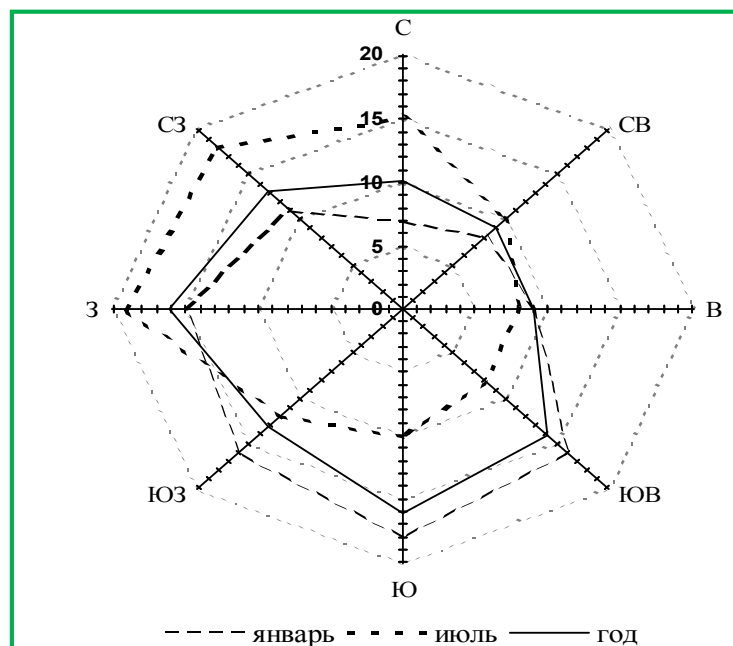
Рисунок 3.2- Роза ветров для метеостанции «Могилев» по данным многолетних наблюдений
