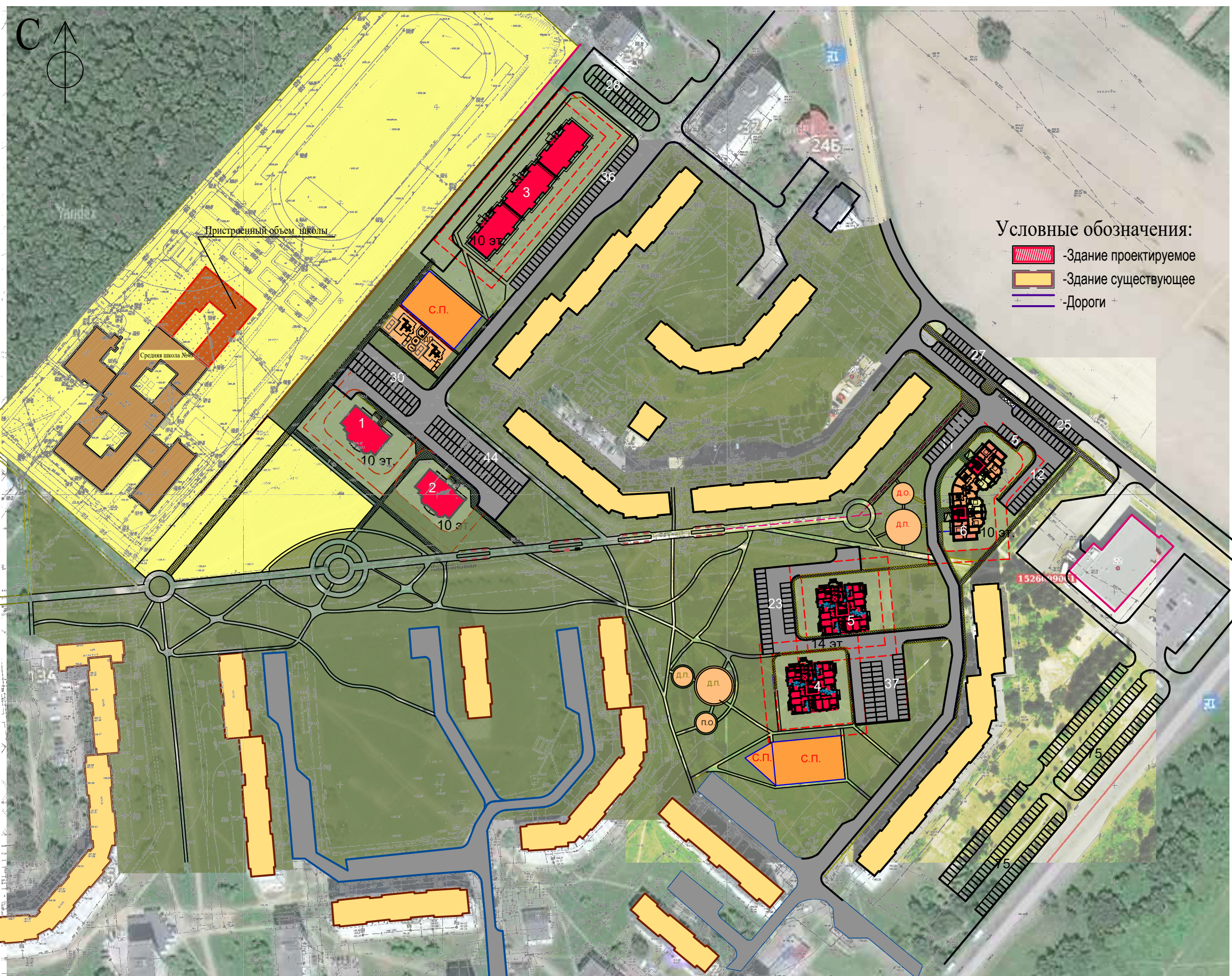
Схема генерального плана
